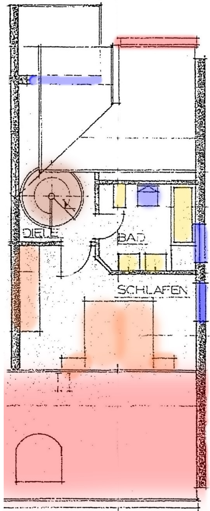
Grundriss 2. DG
