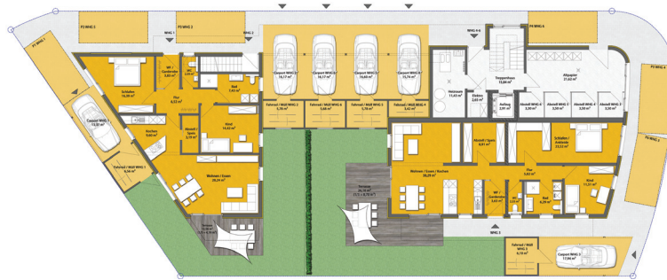
Ergeschoß
